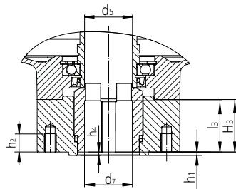
Abtriebsform B1, B2, B Steckbuchse *
