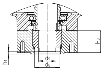
Abtriebsform C Klauenkupplung *
