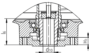
Abtriebsform B3, B4, E Bohrung *
